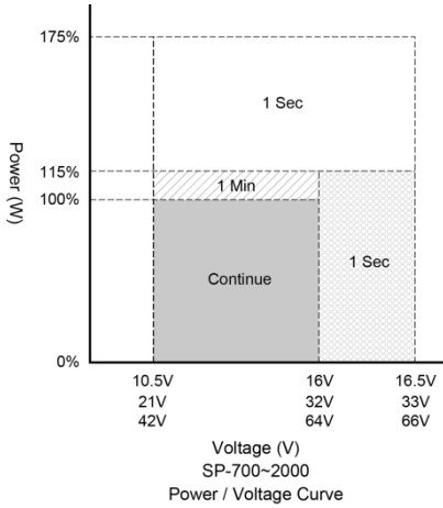
Schéma 1 – SP-700~SP-2000 Puissance en sortie / Tension d'alimentation
